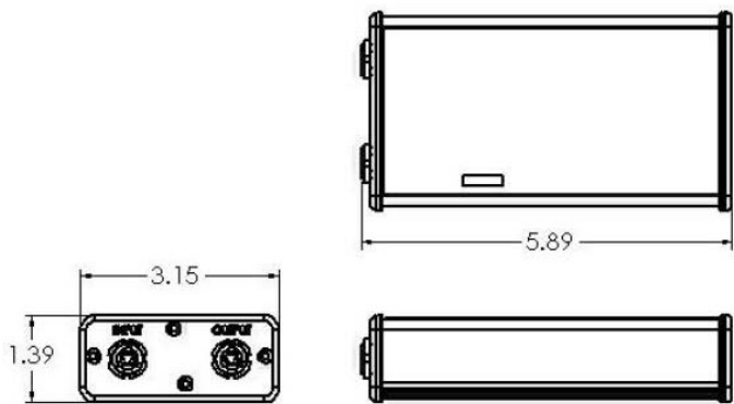
CHARGER MODULE (CH0011)
